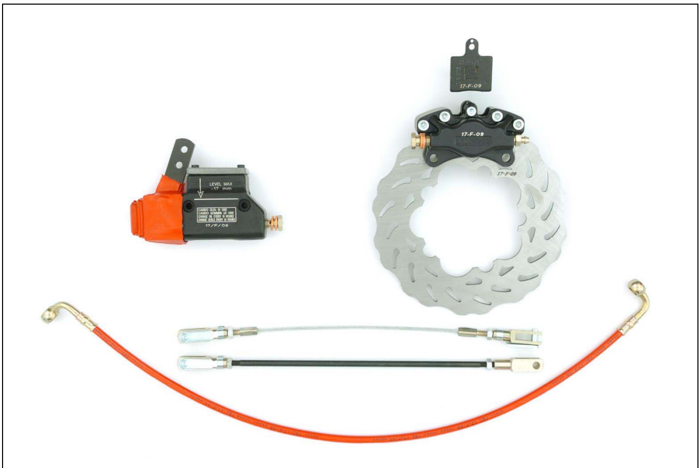
FOTO DEL SISTEMA FRENANTE COMPLETO
